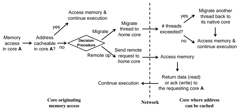
Figure 3: The life of a memory access under EM 2 -RA.
